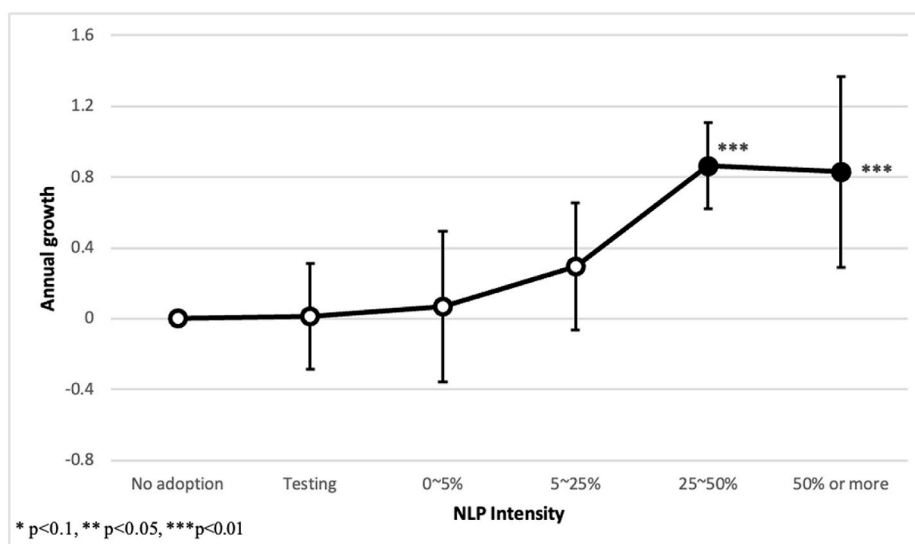
Fig. 1b. Nlp.
