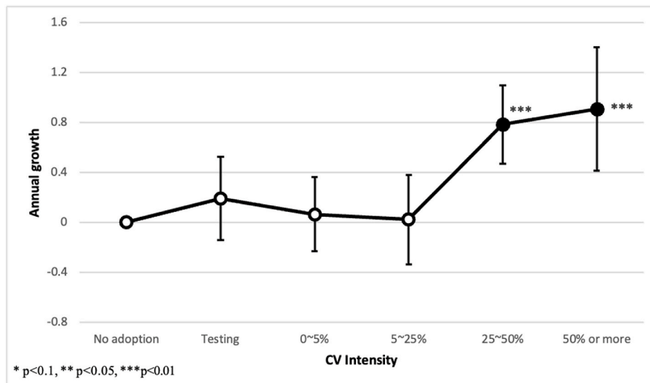
Fig. 1c. CV.
